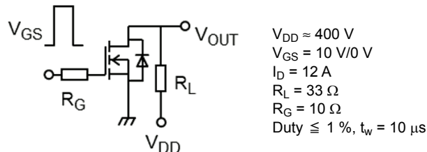
図 6.2.1 スwitching時間の測定回路
