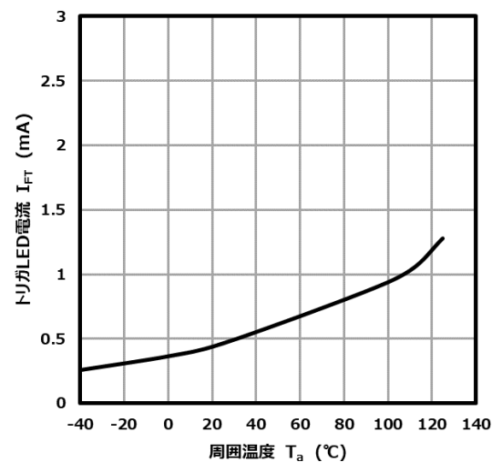
図 12.4 I_{FT} - T_a
