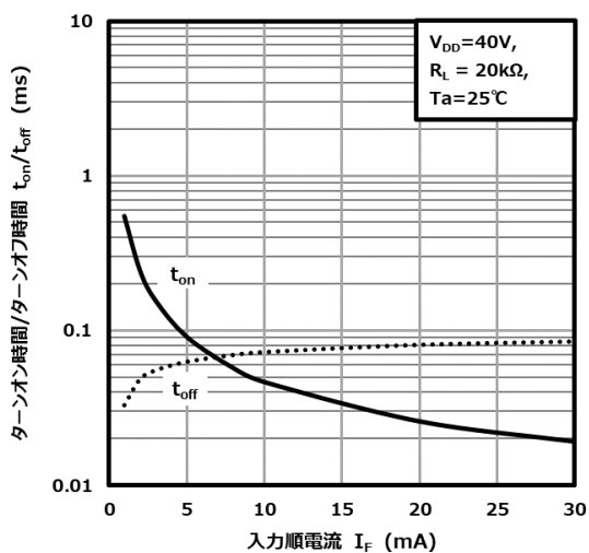
図 12.8 t_{ON}/t_{OFF} - I_F
