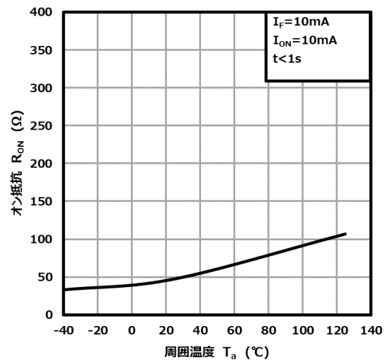
図 12.6 R_{ON} - T_a
