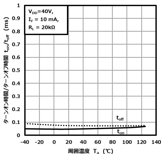
図 12.9 t_{ON}/t_{OFF} - T_a
