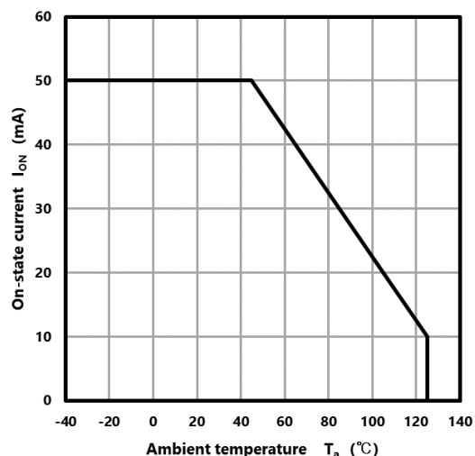
Fig. 12.2 I_{ON} - T_a
