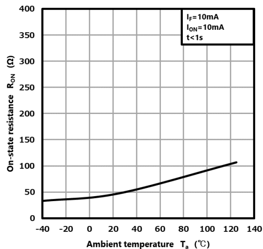
Fig. 12.6 R_{ON} - T_a
