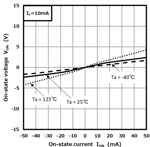
Fig. 12.5 V_{ON} - I_{ON}
