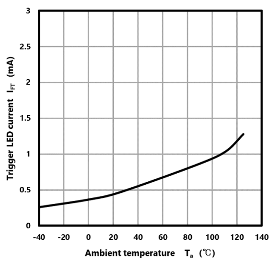
Fig. 12.4 I_{FT} - T_a
