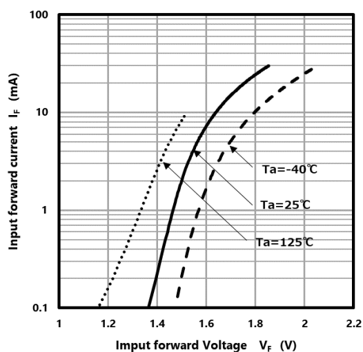
Fig. 12.3 I_F - V_F
