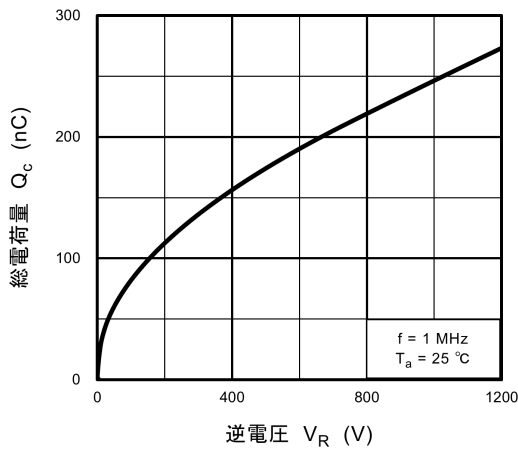
図 9.5 Q_c - V_R
