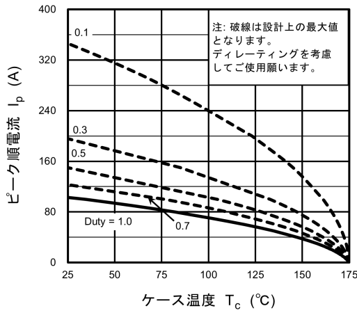
図 9.7 I_p - T_c
