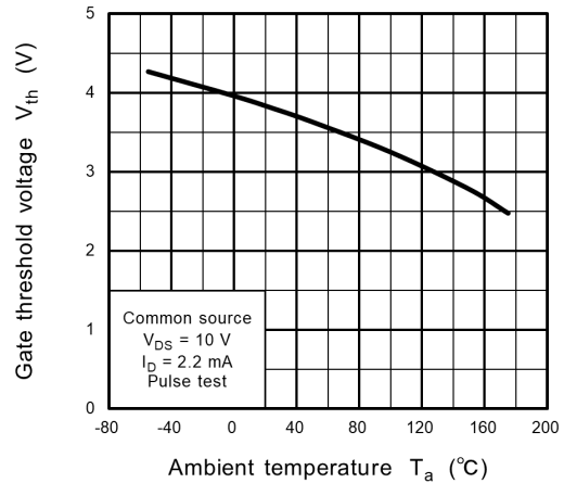
Fig. 8.8 V_{th} - T_a
