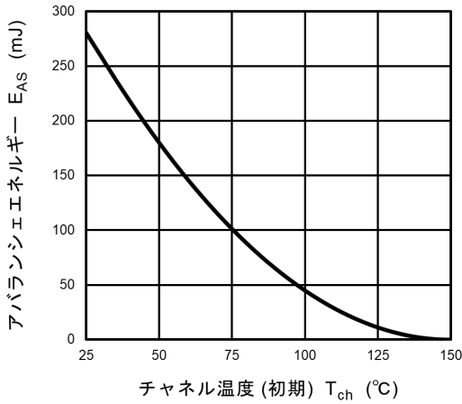
アバラシエエネルギー E_{AS} (mJ) チャネル温度 (初期) T_{ch} (°C) 図 8.14 E_{AS} - T_{ch} (最大値 (保証値))
