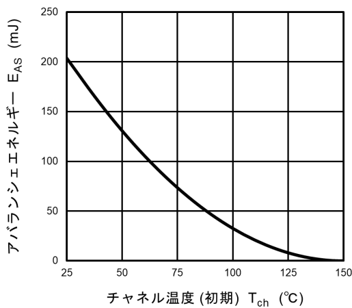
アバラシエエエネルギー E_{AS} (mJ) チャネル温度 (初期) T_{ch} (°C) 図 8.14 E_{AS} - T_{ch} (最大値 (保証値))
