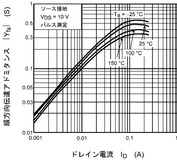
図 7.8 |Y_{fs}| - I_D
