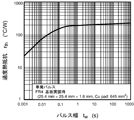
図 7.13 r_{th} - t_w
