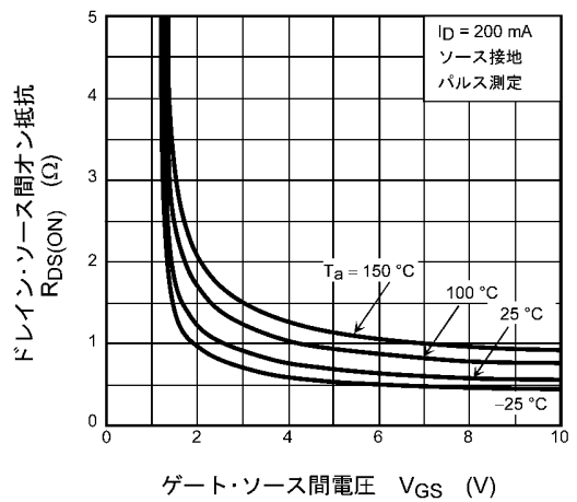
図 7.4 R_{DS(ON)} - V_{GS}
