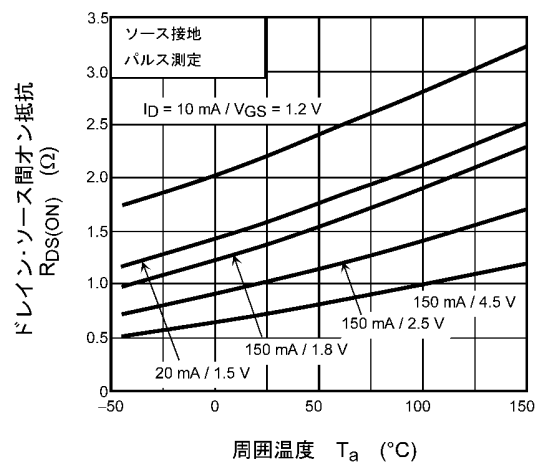
図 7.6 R_{DS(ON)} - T_a
