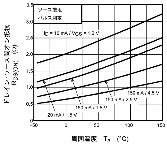
図 7.6 R_{DS(ON)} - T_a
