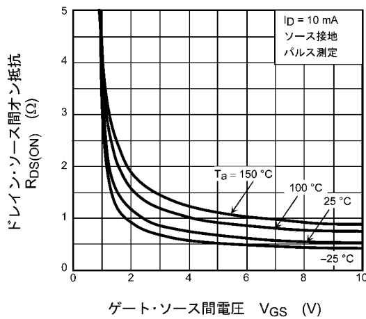
図 7.3 R_{DS(ON)} - V_{GS}
