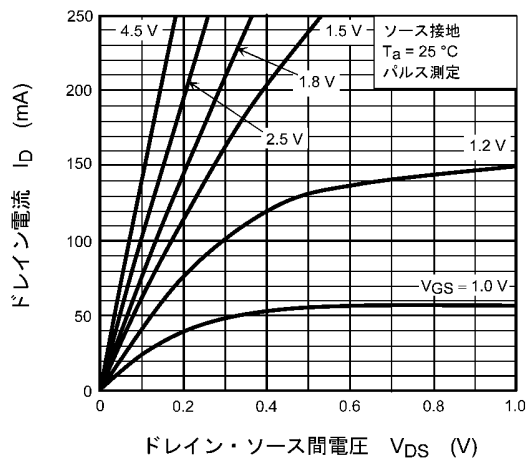
図 7.1 I_D - V_{DS}
