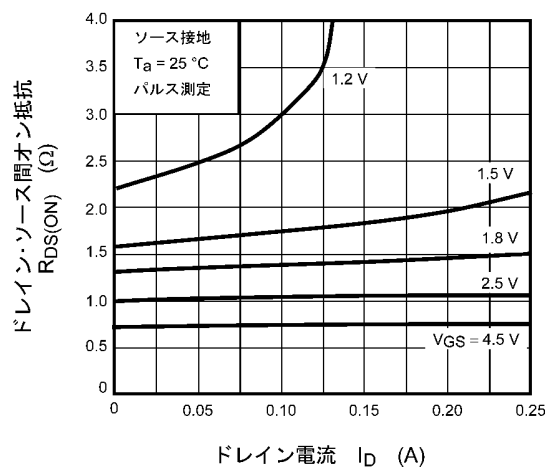
図 7.5 R_{DS(ON)} - I_D
