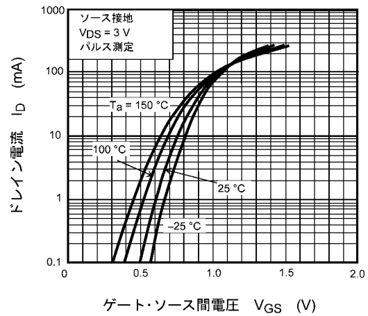
図 7.2 I_D - V_{GS}
