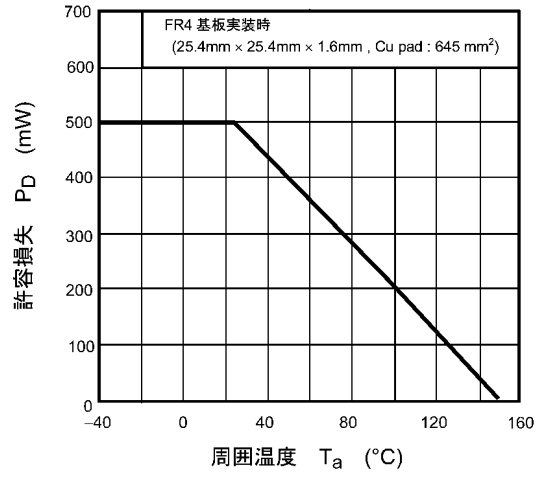
図 7.14 P_D - T_a
