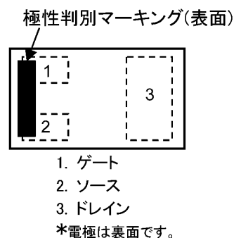
図 6.2 ピン配置 (Top View)
