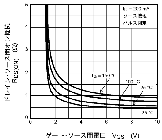
図 7.4 R_{DS(ON)} - V_{GS}
