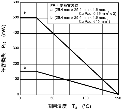
图 7.13 P_D - T_a
