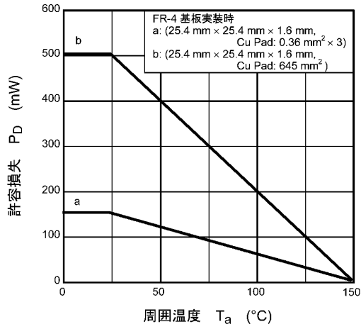
図 7.13 P_D - T_a
