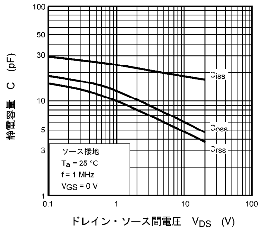
図 7.10 C - V_{DS}
