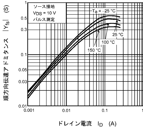
図 7.8 |Y_{fs}| - I_D
