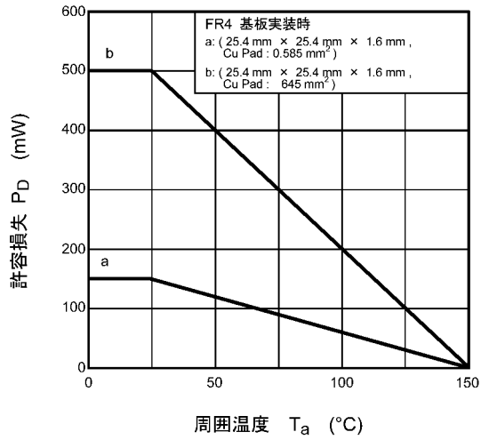
図 7.13 P_D - T_a
