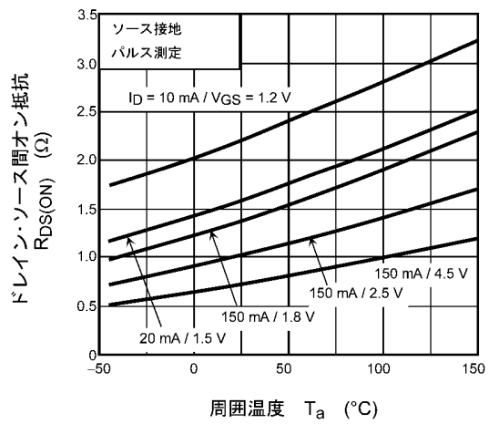
図 7.6 R_{DS(ON)} - T_a
