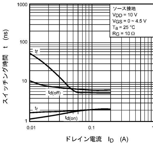
図 7.11 t - I_D
