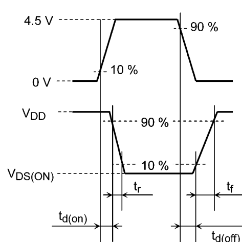
図 5.3.2 入力波形/出力波形
