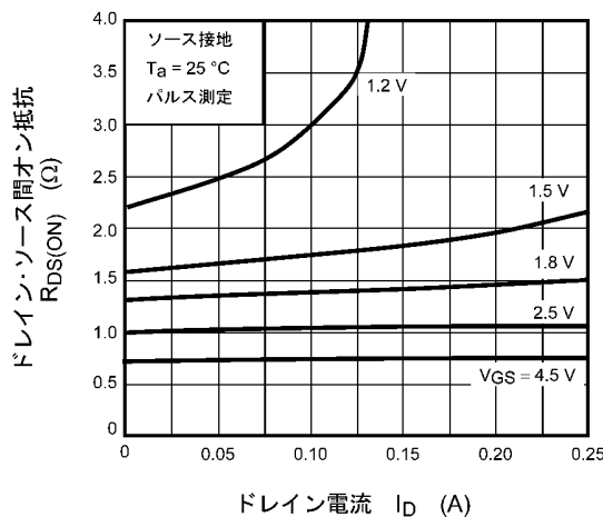
図 7.5 R_{DS(ON)} - I_D
