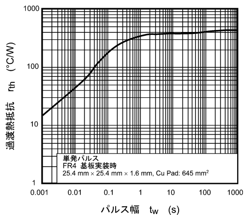
図 7.13 r_{th} - t_w
