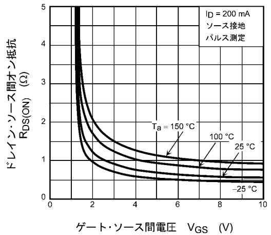
図 7.4 R_{DS(ON)} - V_{GS}
