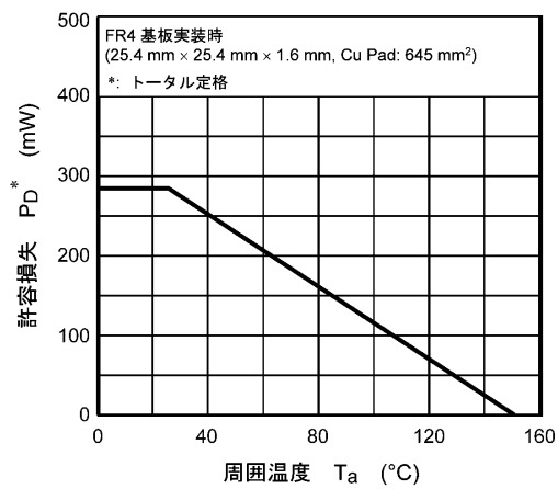
図 7.14 P_D - T_a
