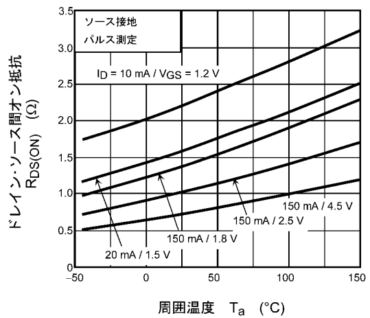
図 7.6 R_{DS(ON)} - T_a
