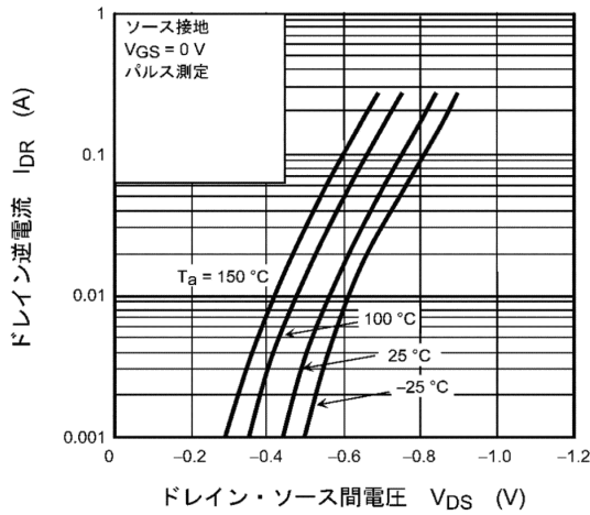
図 7.9 I_{DR} - V_{DS}
