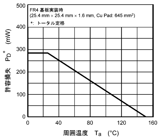
図 7.14 P_D - T_a
