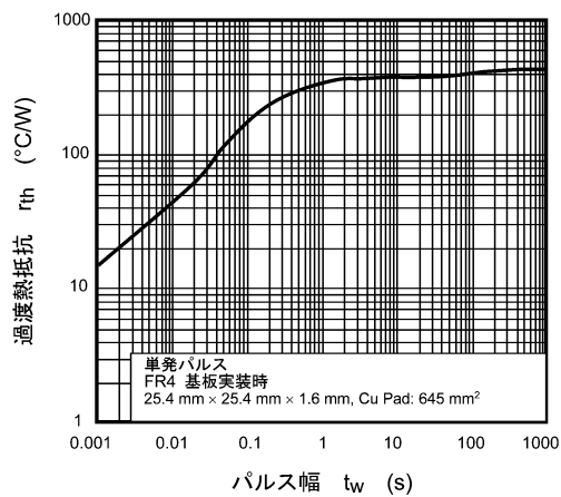
図 7.13 r_{th} - t_w
