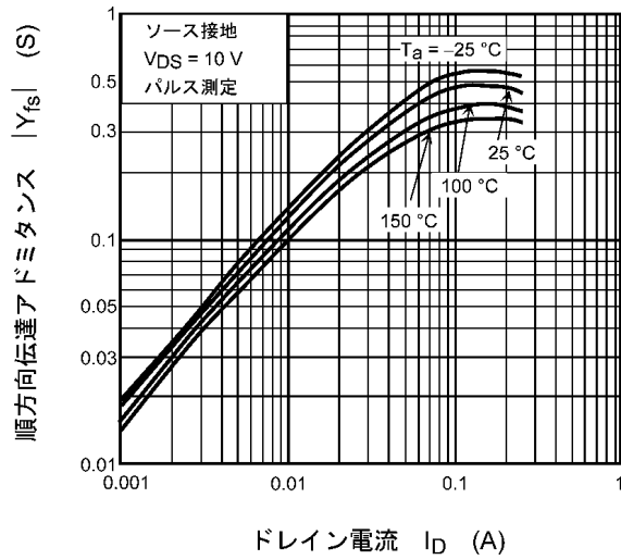
図 7.8 |Y_{fs}| - I_D
