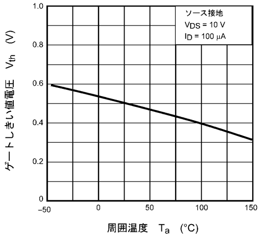
図 7.7 V_{th} - T_a
