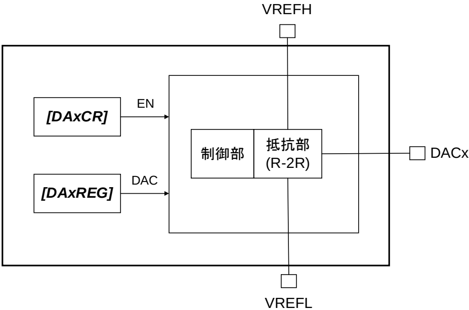
図 2.1 8ビットデジタルアナログコンバーターブロック図
