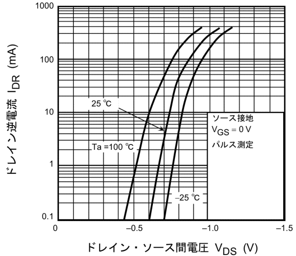
図 8.8 I_{DR} - V_{DS}
