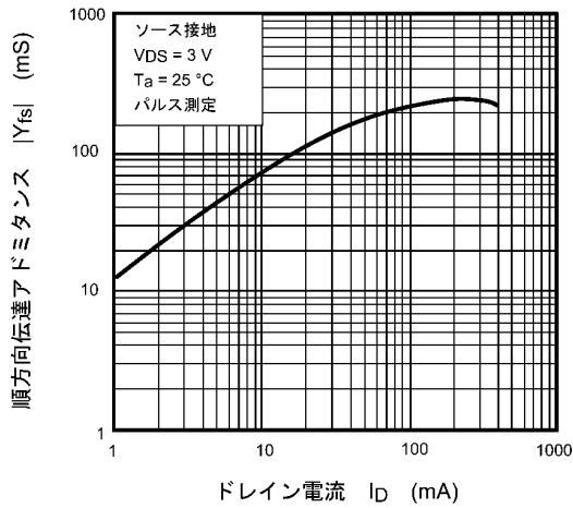
図 8.7 |Y_{fs}| - I_D
