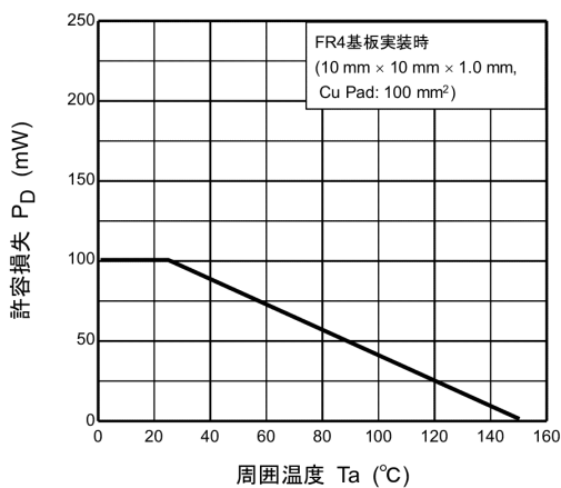
図 8.11 P_D - T_a
