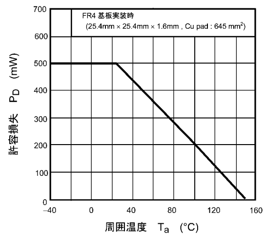
図 8.12 P_D - T_a
