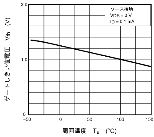
図 8.6 V_{th} - T_a
