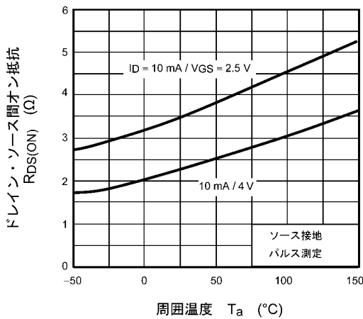
図 8.5 R_{DS(ON)} - T_a
