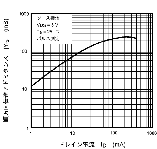
図 8.7 |Y_{fs}| - I_D
