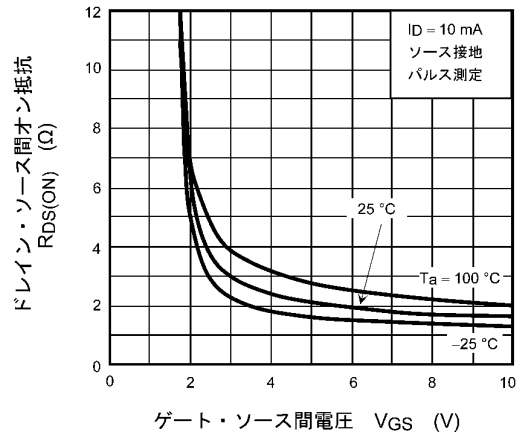
図 8.4 R_{DS(ON)} - V_{GS}
