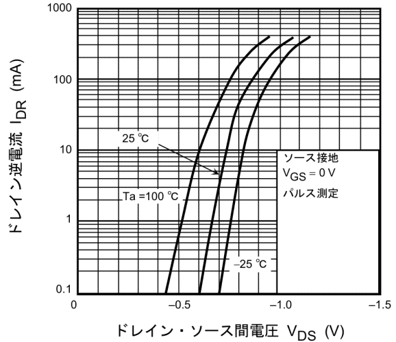
図 8.8 I_{DR} - V_{DS}
