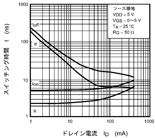
図 8.10 t - I_D
