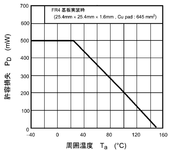
図 8.12 P_D - T_a
