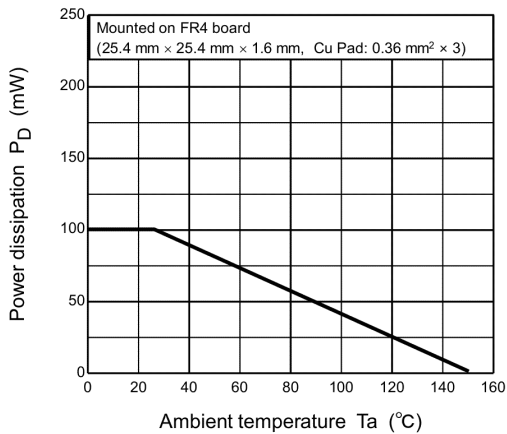
Fig. 7.11 P_D - T_a
