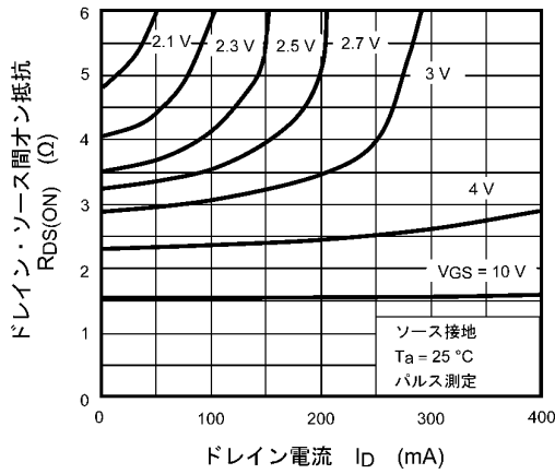
図 7.3 R_{DS(ON)} - I_D
