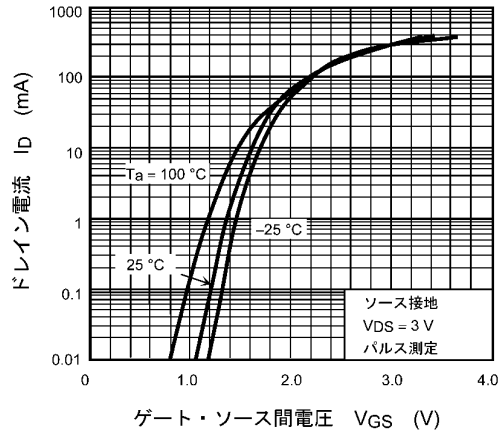
図 7.2 I_D - V_{GS}
