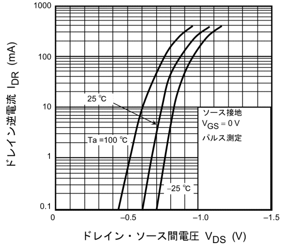
図 7.8 I_{DR} - V_{DS}
