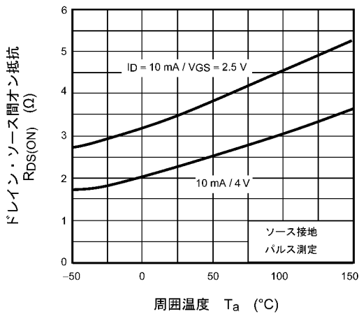
図 7.5 R_{DS(ON)} - T_a
