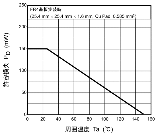
図 7.11 P_D - T_a
