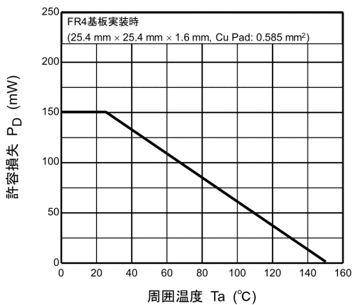
図 7.11 P_D - T_a
