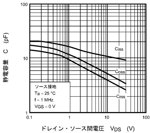
図 7.9 C - V_{DS}
