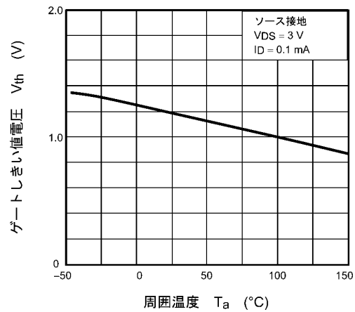
図 7.6 V_{th} - T_a
