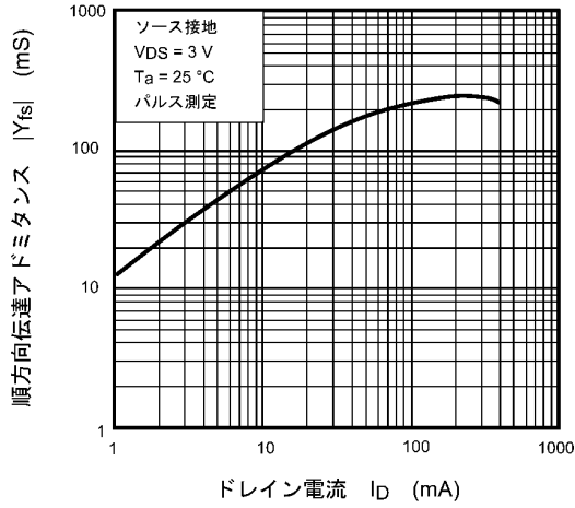
図 7.7 |Y_{fs}| - I_D
