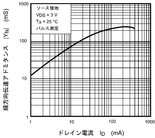
図 7.7 |Y_{fs}| - I_D
