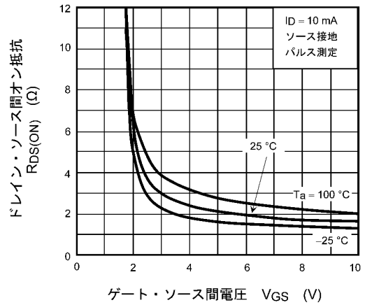
図 7.4 R_{DS(ON)} - V_{GS}
