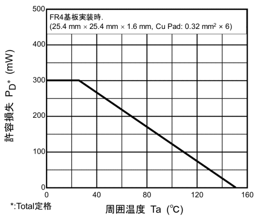
図 7.11 P_D - T_a
