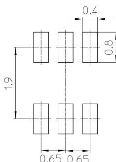
図 4.1 参考パッド寸法 (Unit: mm)
