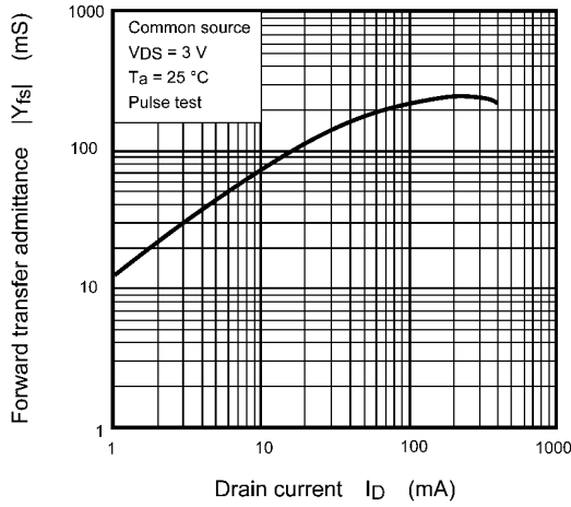
Fig. 8.7 |Y_{fs}| - I_D
