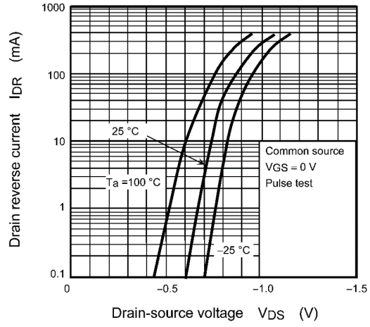
Fig. 8.8 I_{DR} - V_{DS}
