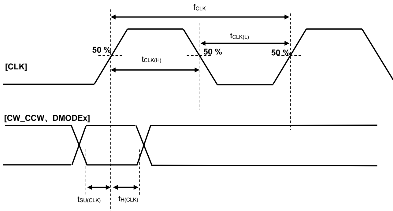
図 20.2 TB67S559FTG(CLK とその他制御信号の関係)
