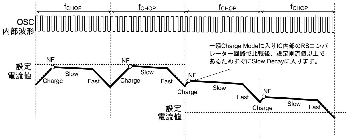
図 7.11.3 設定電流値が減少方向の場合
