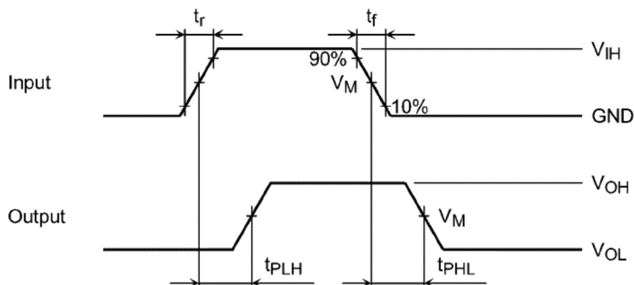
図 9.8.1 t_{PLH} , t_{PHL}
