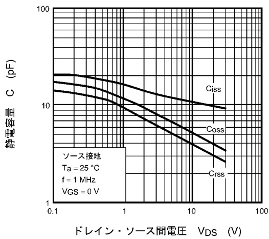
図 7.9 C - V_{DS}
