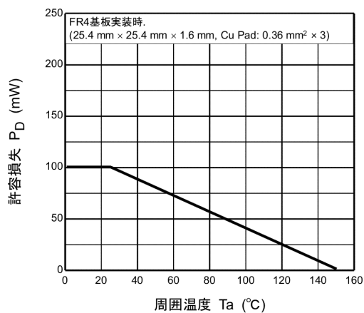
図 7.11 P_D - T_a
