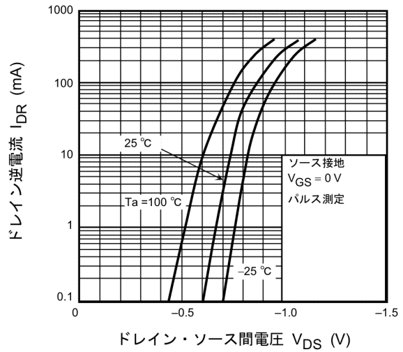
図 7.8 I_{DR} - V_{DS}
