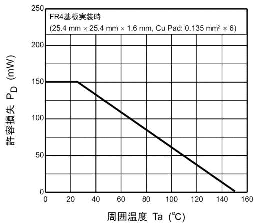
図 7.11 P_D - T_a
