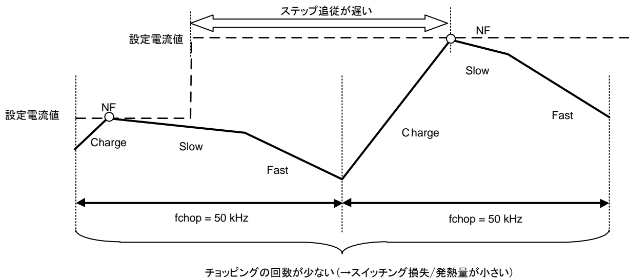
図 4.3 定電流波形 (fchop = 50 kHz の場合)
