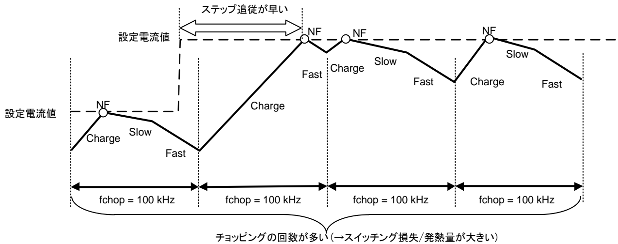
図 4.2 定電流波形 (fchop = 100 kHz の場合)
