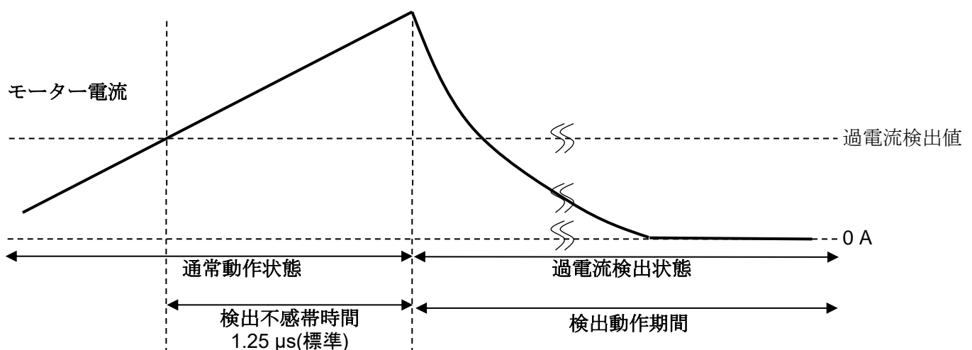
図 5.2 ISD 動作
