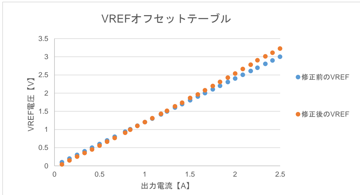
図 4.1 VREF オフセットテーブル
