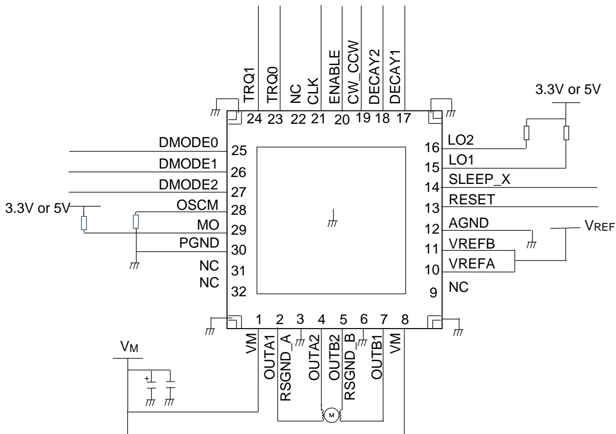
図 7.1 応用回路例
