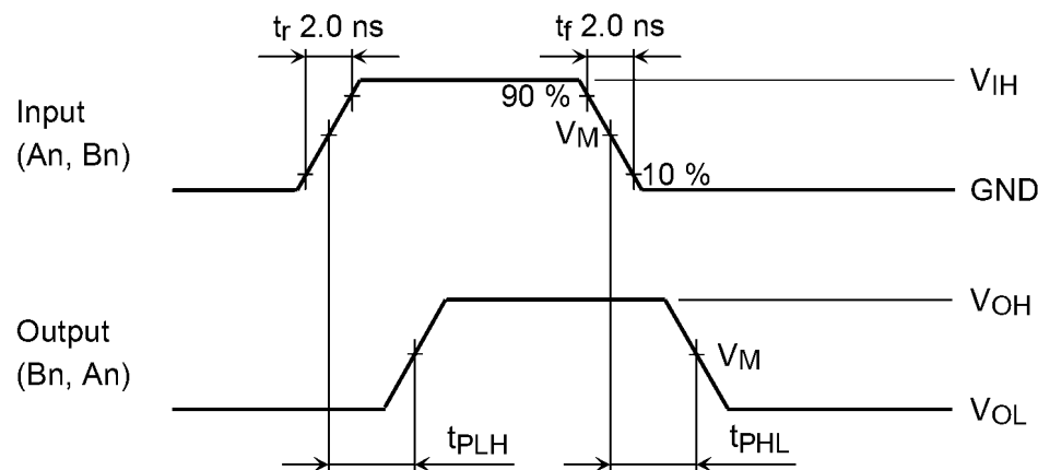
図 13.1 tPLH, tPHL
