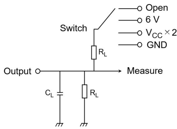
図 12.1 AC電氣の特性測定回路
