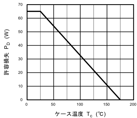
ケース温度 T_c (°C) 図 8.16 P_D - T_c (最大値 (保証値))
