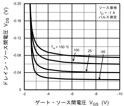
図 8.6 V_{DS} - V_{GS}
