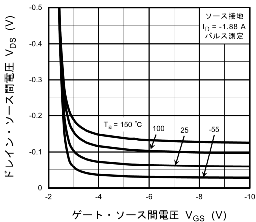
図 8.5 V_{DS} - V_{GS}
