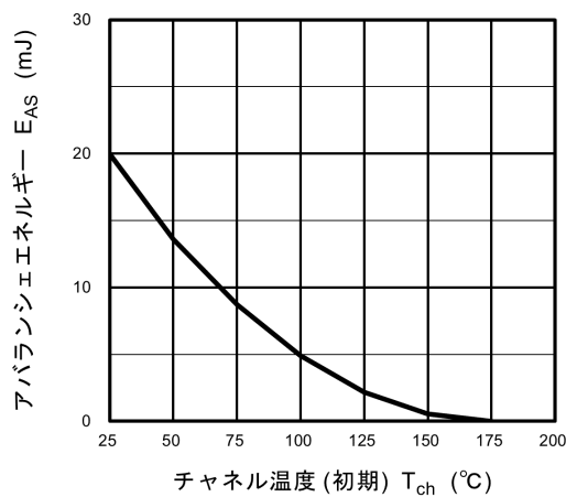
チャンネル温度 (初期) T_{ch} (°C) 図 8.15 E_{AS} - T_{ch}
