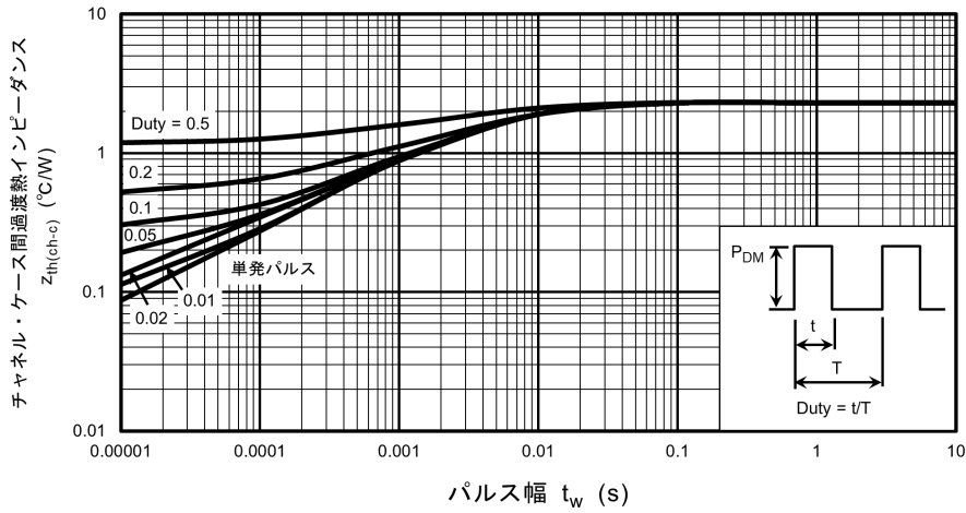
図 8.18 Z_{th(ch-c)} - t_w (最大値 (保証値))
