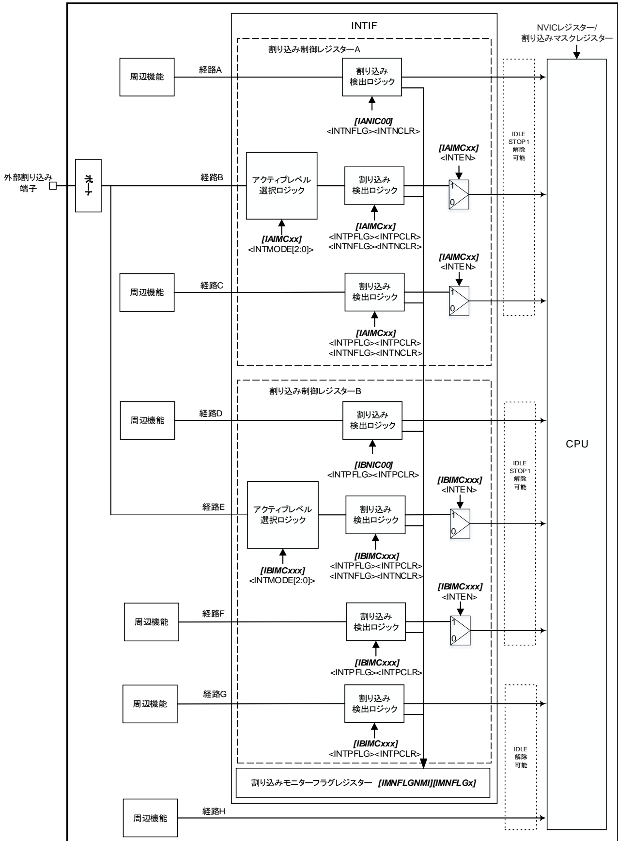
図 4.1 割り込み伝達経路
