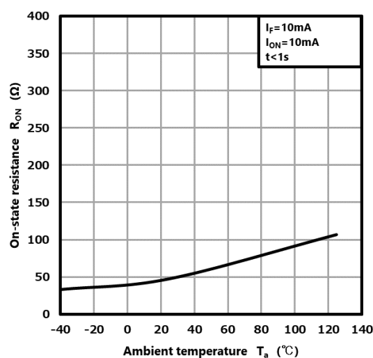
Fig. 12.6 R_{ON} - T_a
