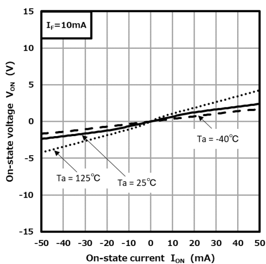
Fig. 12.5 V_{ON} - I_{ON}
