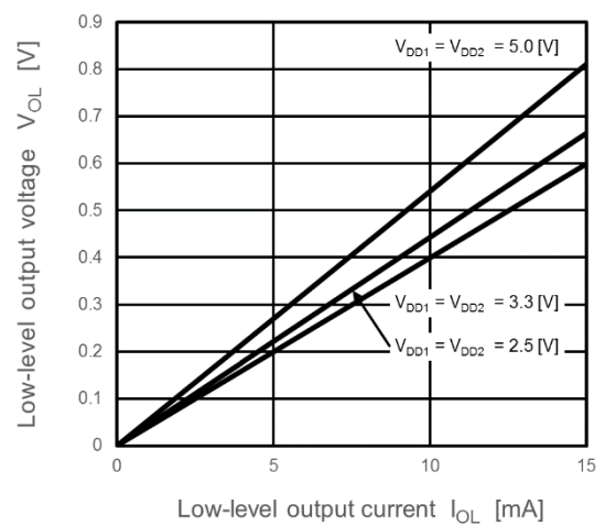
Fig.13.6 VOL-IOL
