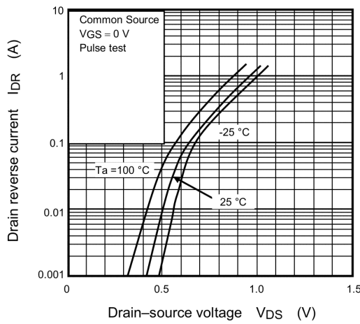
Fig. 7.9 I_{DR} - V_{DS}
