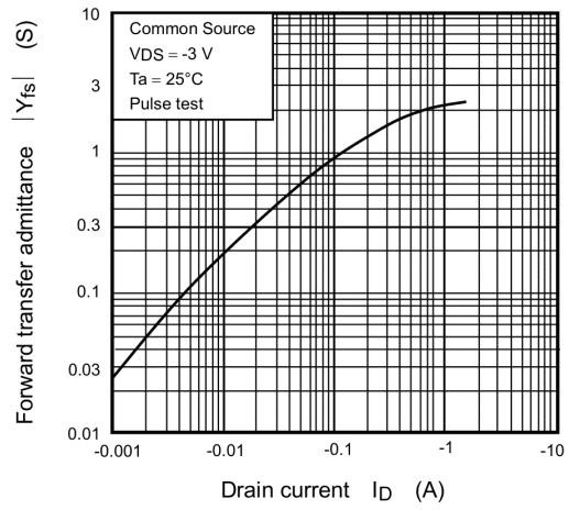
Fig. 7.8 |Y_{fs}| - I_D
