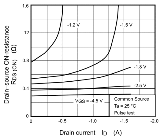
Fig. 7.6 R_{DS(ON)} - I_D
