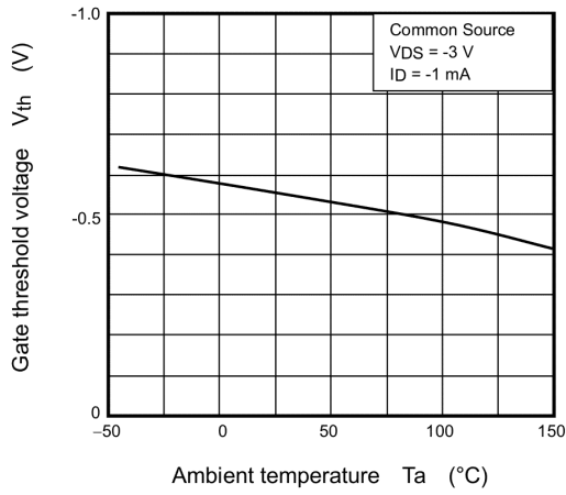
Fig. 7.7 V_{th} - T_a
