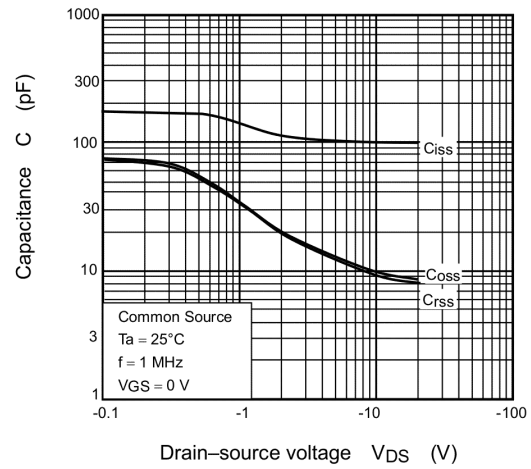
Fig. 7.10 C - V_{DS}
