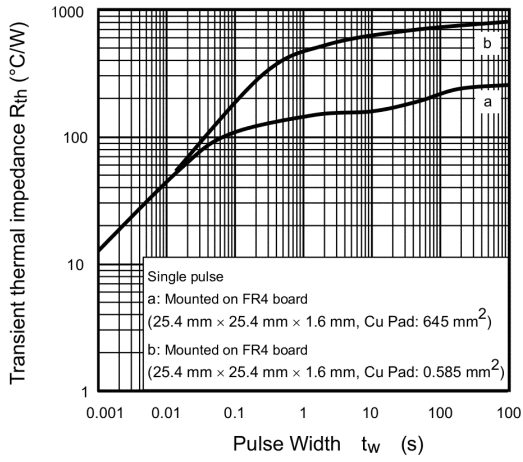
Fig. 7.13 r_{th} - t_w
