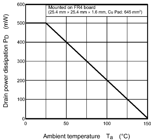
Fig. 9.11 P_D - T_a
