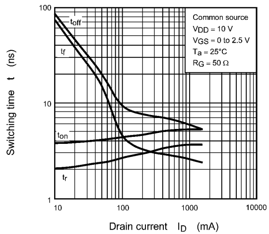
Fig. 7.10 t - I_D
