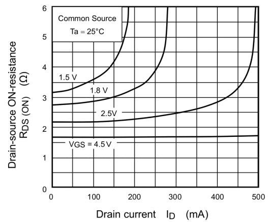
Fig. 7.4 R_{DS(ON)} - I_D
