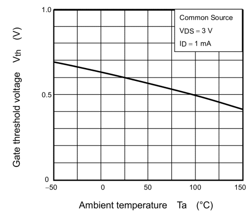
Fig. 7.6 V_{th} - T_a
