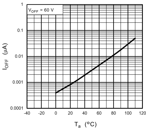
図 12.1.9 I_{OFF} - T_a
