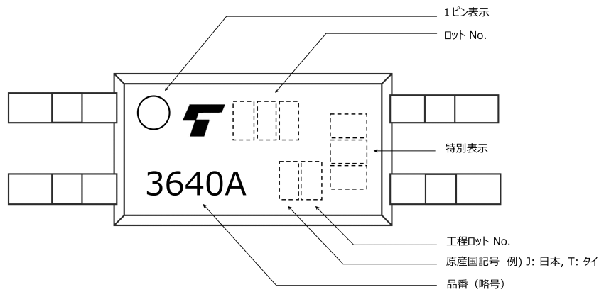
図 15.1 TLP3640A 現品表示
