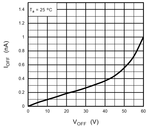
図 12.1.10 I_{OFF} - V_{OFF}
