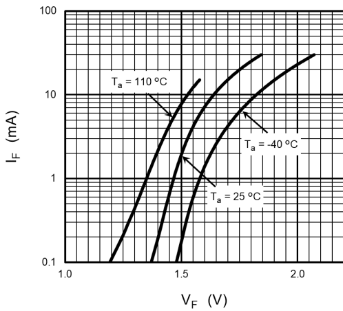
図 12.1.3 I_F - V_F
