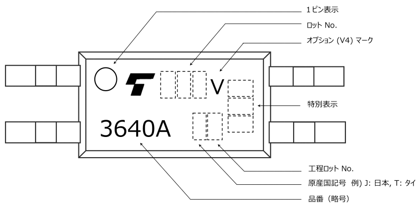
図 17.3 TLP3640A(オプション "V4" 品)現品表示例 (注)
