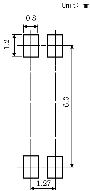
図 14.1 TLP3640A 参考パッド寸法図
