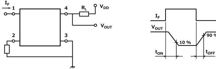
図 10.1 スイッチング時間測定回路, 波形
