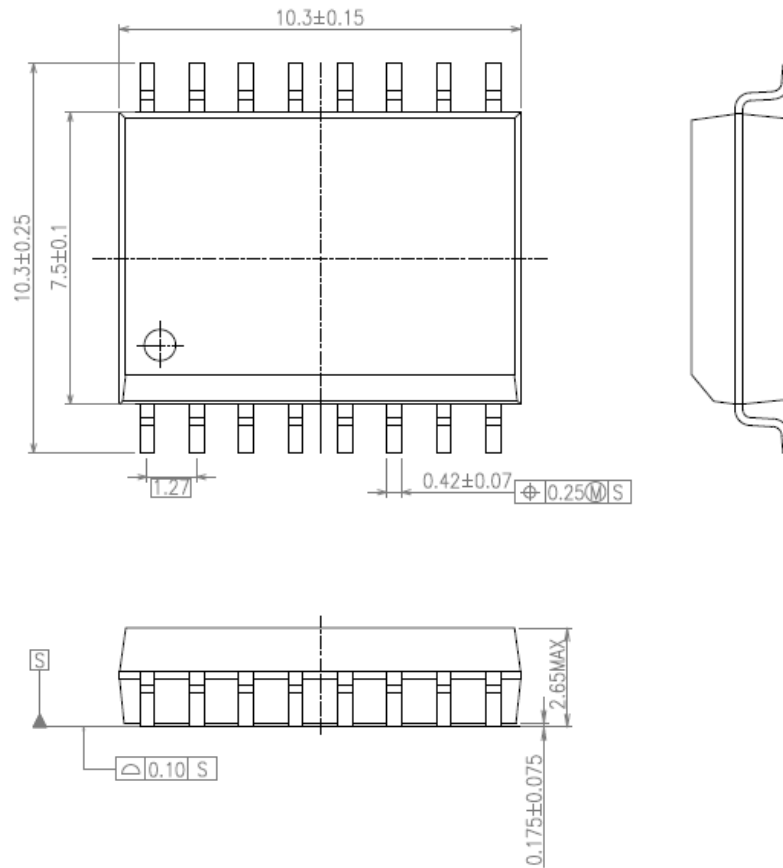
图 14.1 外形寸法图
