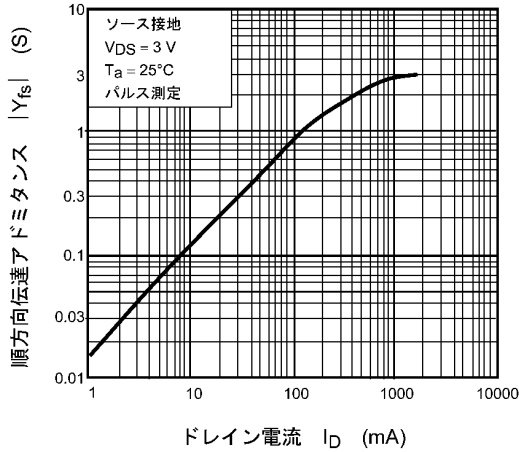
図 7.7 |Y_{fs}| - I_D
