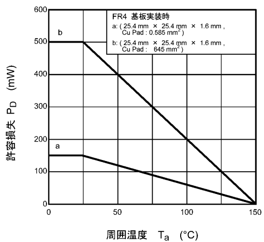
図 7.12 P_D - T_a
