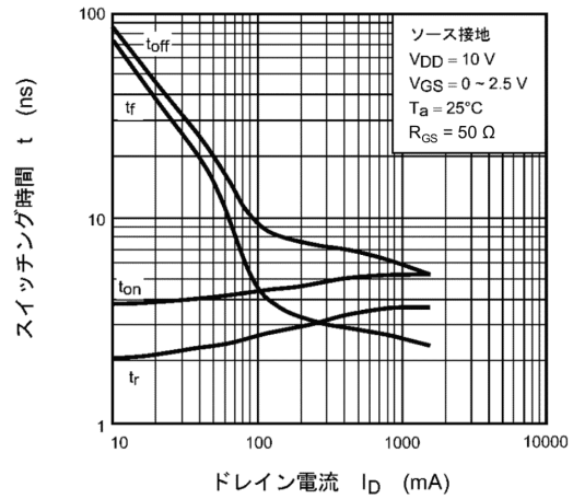
図 7.10 t - I_D
