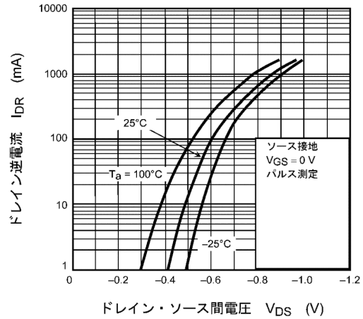
図 7.8 I_{DR} - V_{DS}
