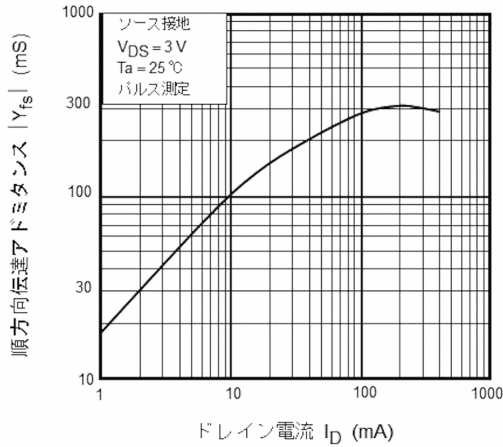
図 7.7 |Y_{fs}| - I_D
