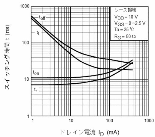
図 7.10 t - I_D
