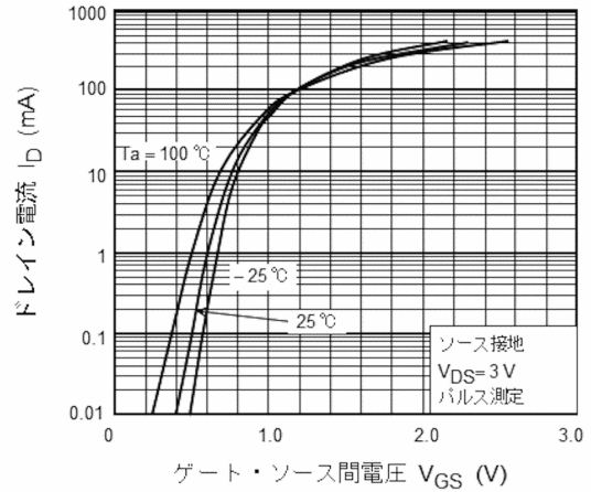
図 7.2 I_D - V_{GS}
