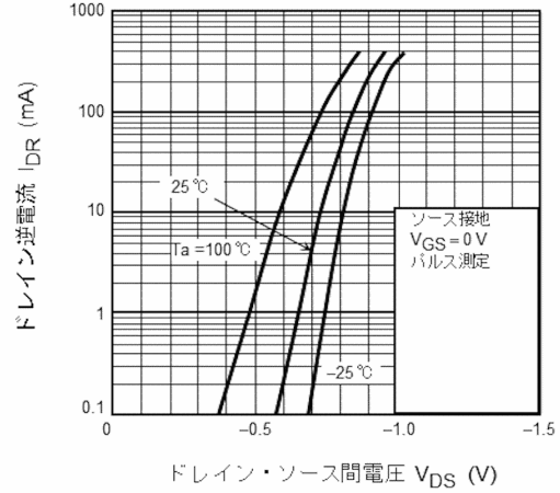
図 7.8 I_{DR} - V_{DS}
