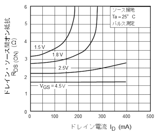
図 7.4 R_{DS(ON)} - I_D
