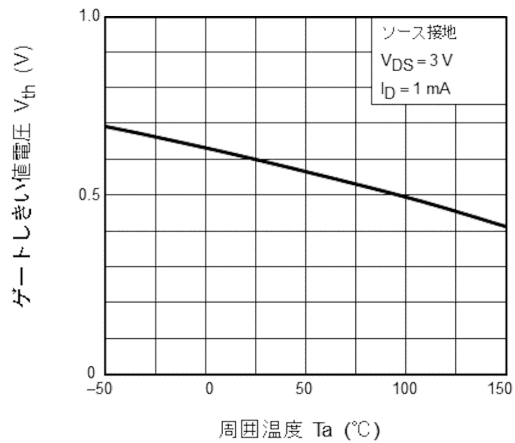
図 7.6 V_{th} - T_a
