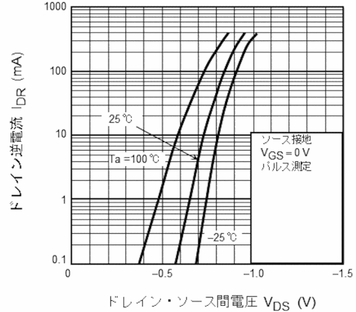
図 7.8 I_{DR} - V_{DS}
