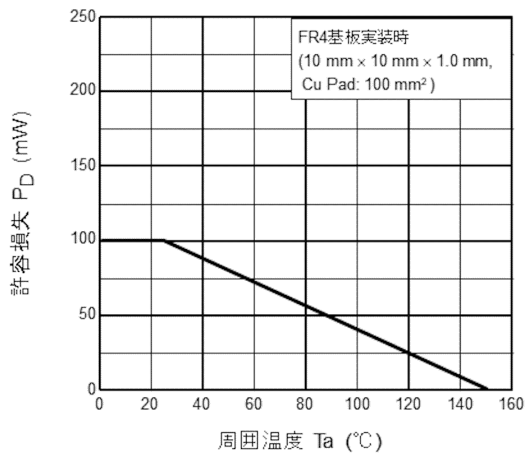
図 7.11 P_D - T_a
