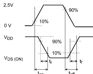
図 5.3.2 入力波形/出力波形
