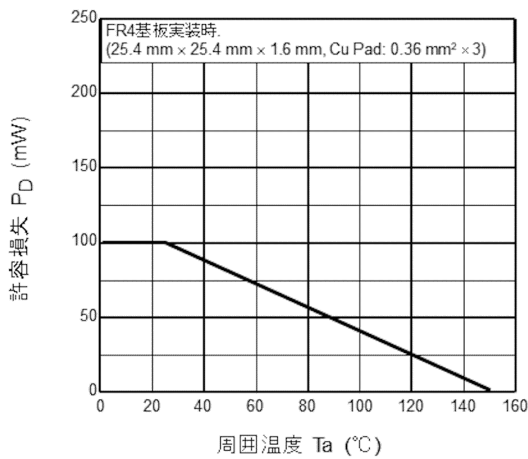
図 7.11 P_D - T_a
