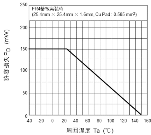
図 7.11 P_D - T_a
