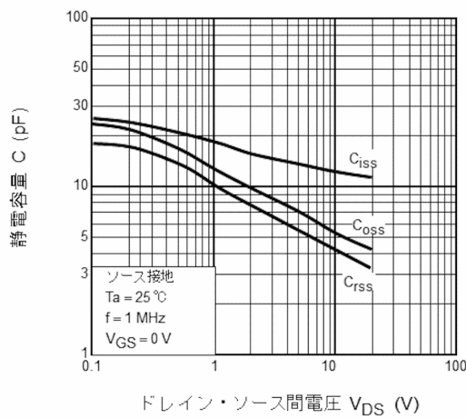
図 7.9 C - V_{DS}
