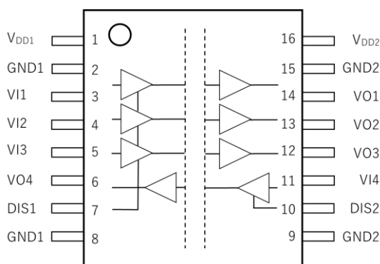
図 6.1 端子配置図 (top view)
