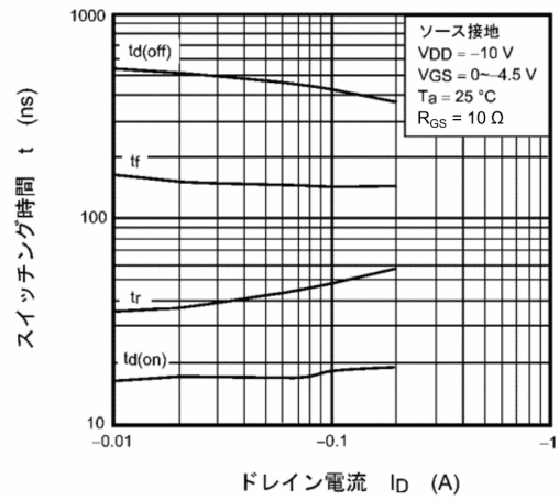
図 9.10 t - I_D
