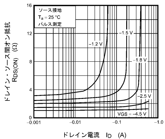
図 9.6 R_{DS(ON)} - I_D
