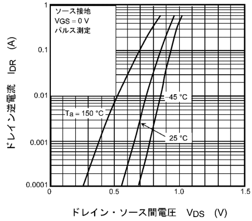
図 9.8 I_{DR} - V_{DS}
