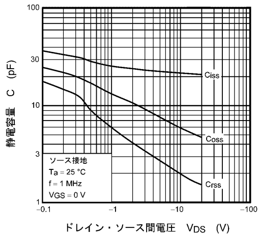
図 9.9 C - V_{DS}
