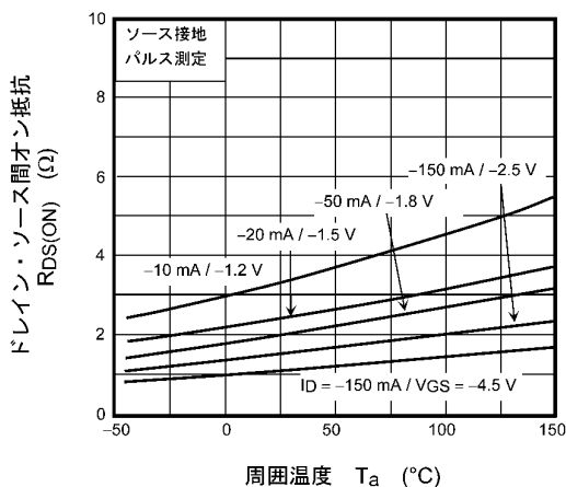
図 9.5 R_{DS(ON)} - T_a
