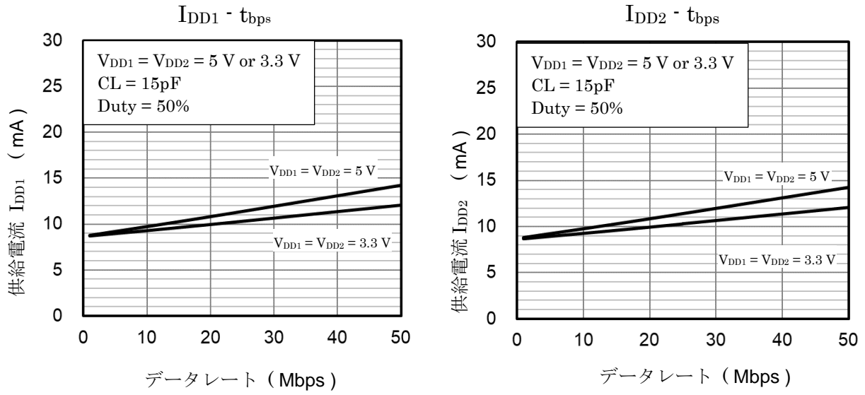
図 12.1 供給電流 - データレート
