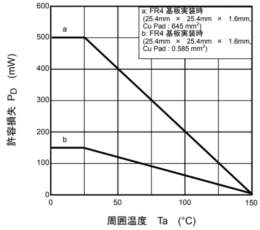
図 7.14 P_D - T_a
