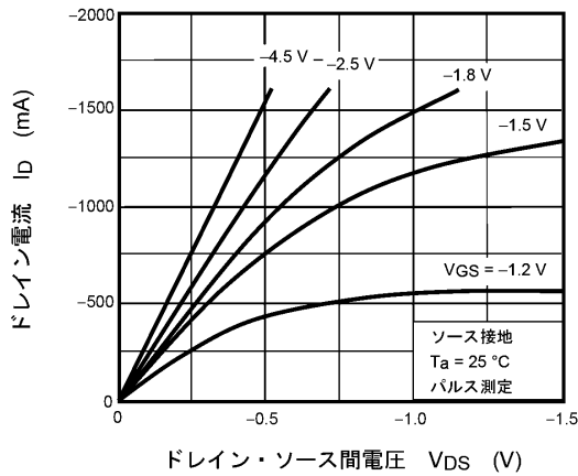
図 7.1 I_D - V_{DS}
