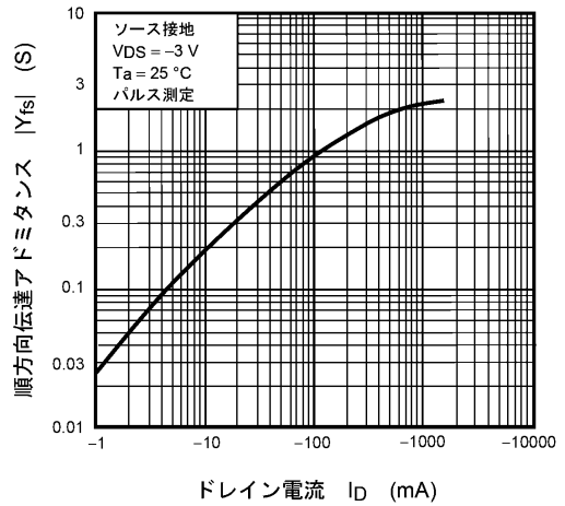
図 7.8 |Y_{fs}| - I_D
