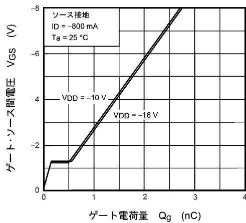
図 7.12 ダイナミック入力特性
