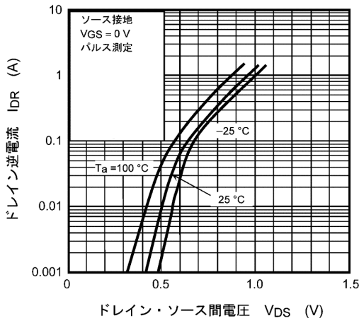
図 7.9 I_{DR} - V_{DS}
