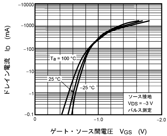
図 7.2 I_D - V_{GS}
