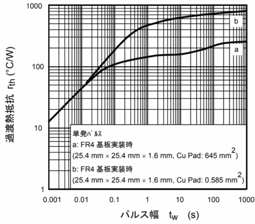
図 7.13 r_{th-t_w}
