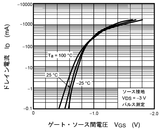
図 7.2 I_D - V_{GS}
