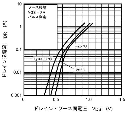
図 7.9 I_{DR} - V_{DS}
