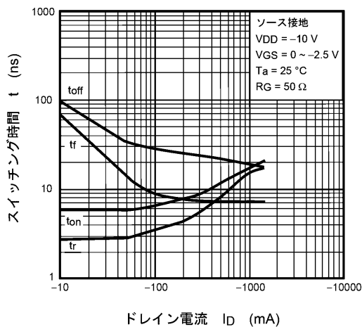
図 7.11 t - I_D
