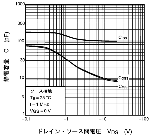
図 7.10 C - V_{DS}
