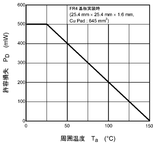
図 8.11 P_D - T_a
