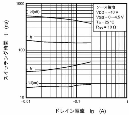
図 8.10 t - I_D
