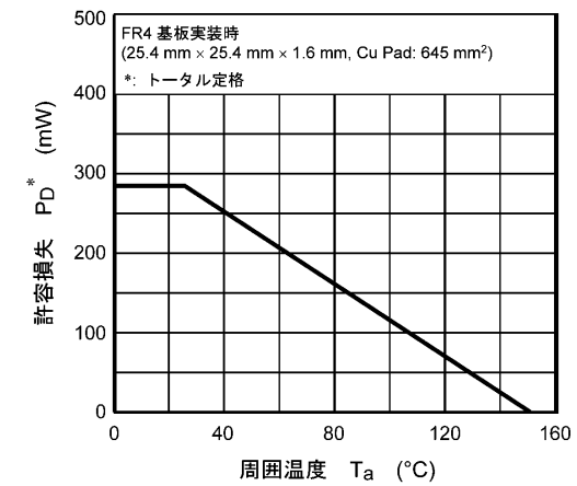
図 8.12 P_D - T_a
