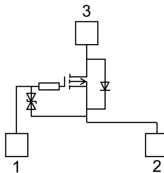
図 7.1 等価回路図
