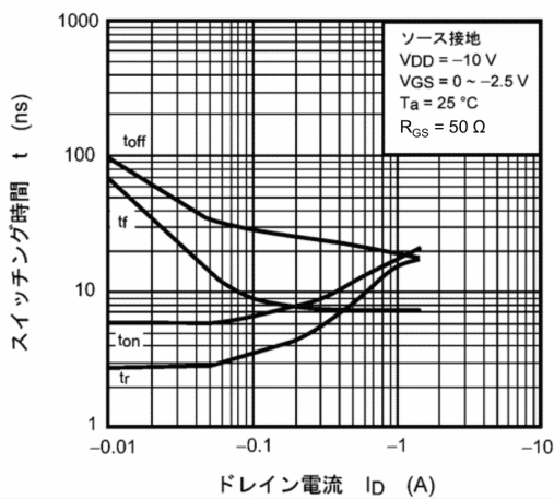
図 8.11 t - I_D
