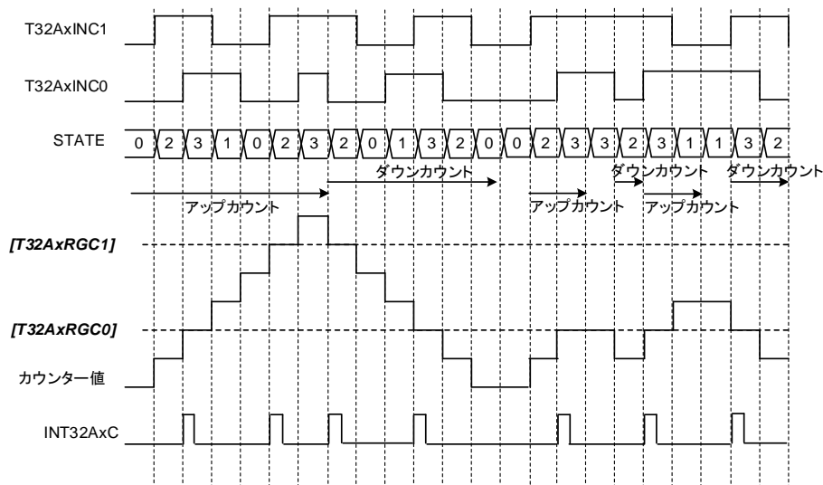
図 3.3 逆位相(<PDIR>=1)時のカウンター動作例
