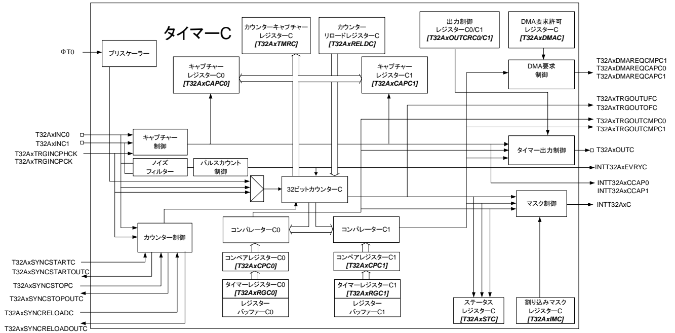
図 2.2 32ビットタイマーブロック図
