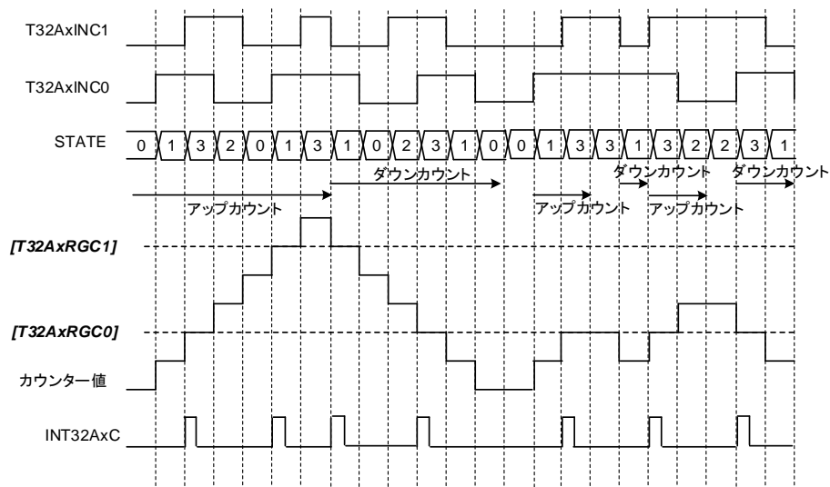
図 3.2 正位相(<PDIR>=0)時のカウンター動作例
