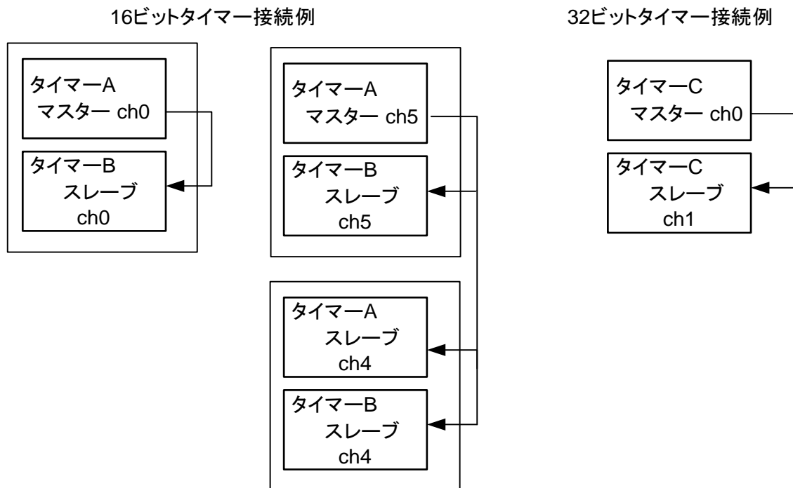
図 3.4 同期動作例
