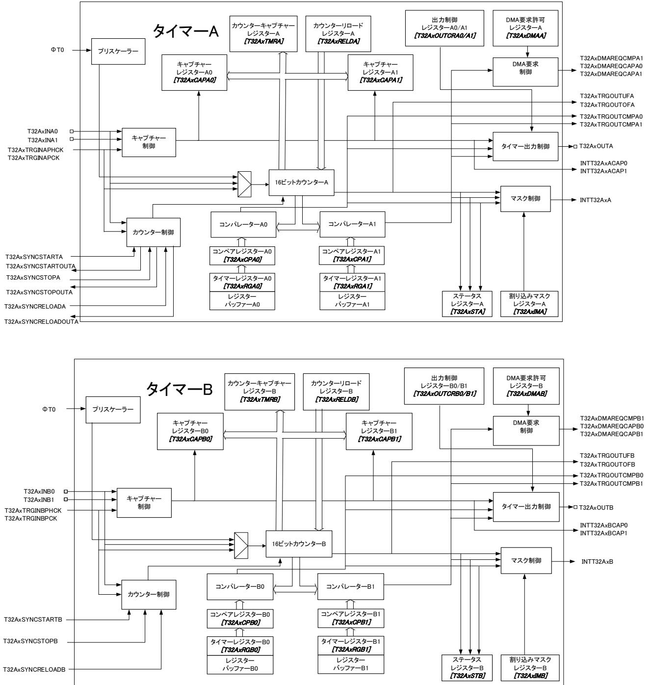
図 2.1 16ビットタイマーブロック図
