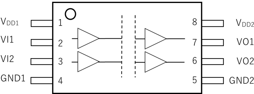
図 6.1 端子配置図 (top view)
