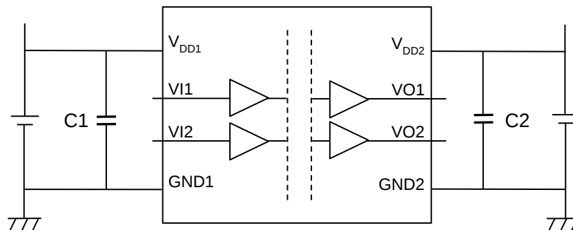
図 8.1 外付け部品回路図 (top view)
