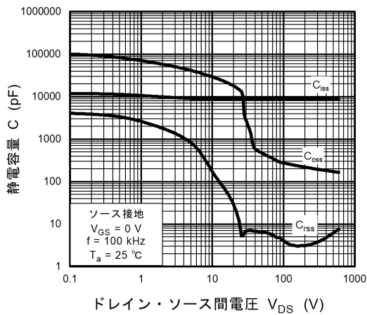
図 8.9 C - V_{DS}
